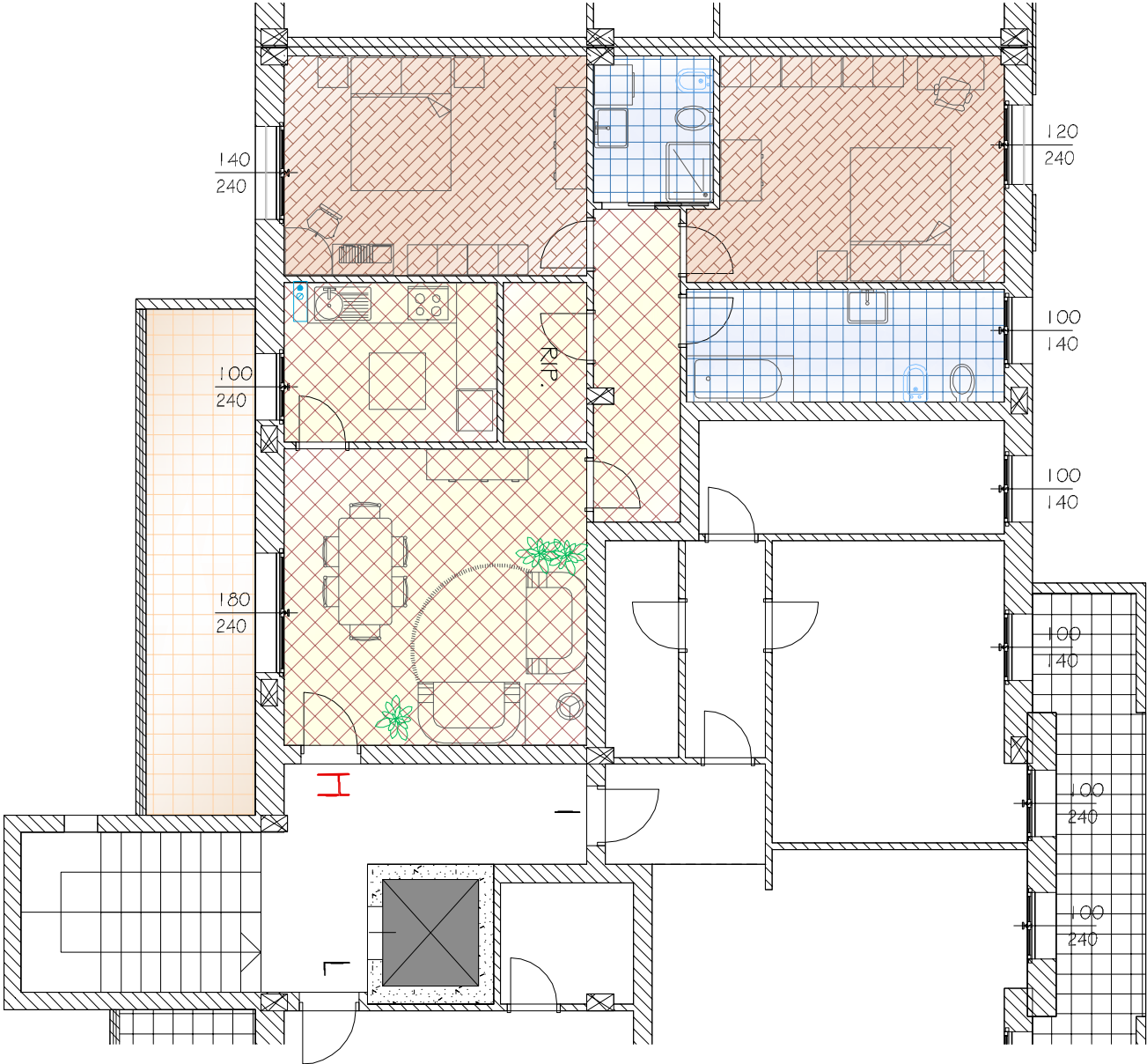
Pianta Arredata
