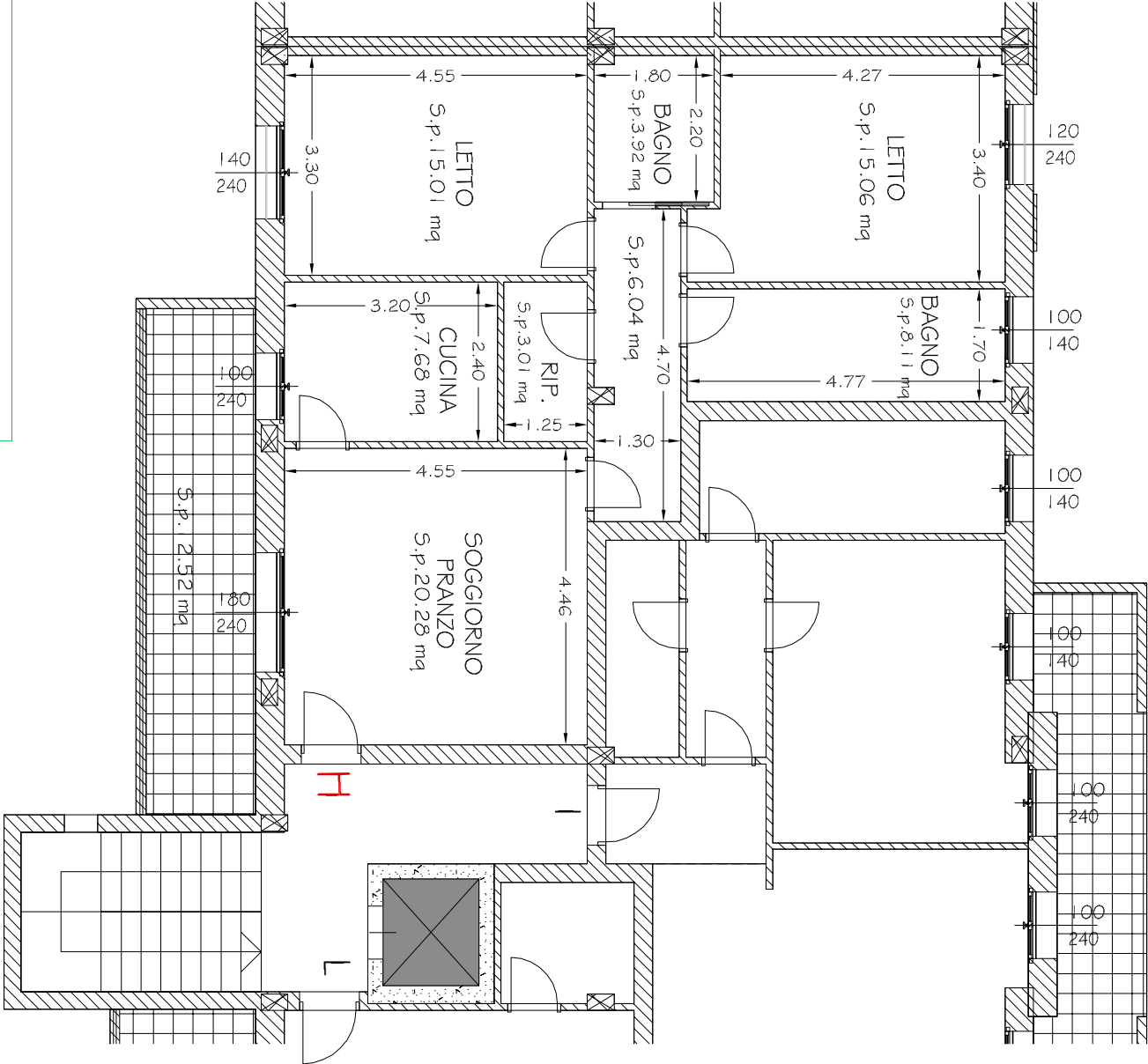
Pianta Quotata
